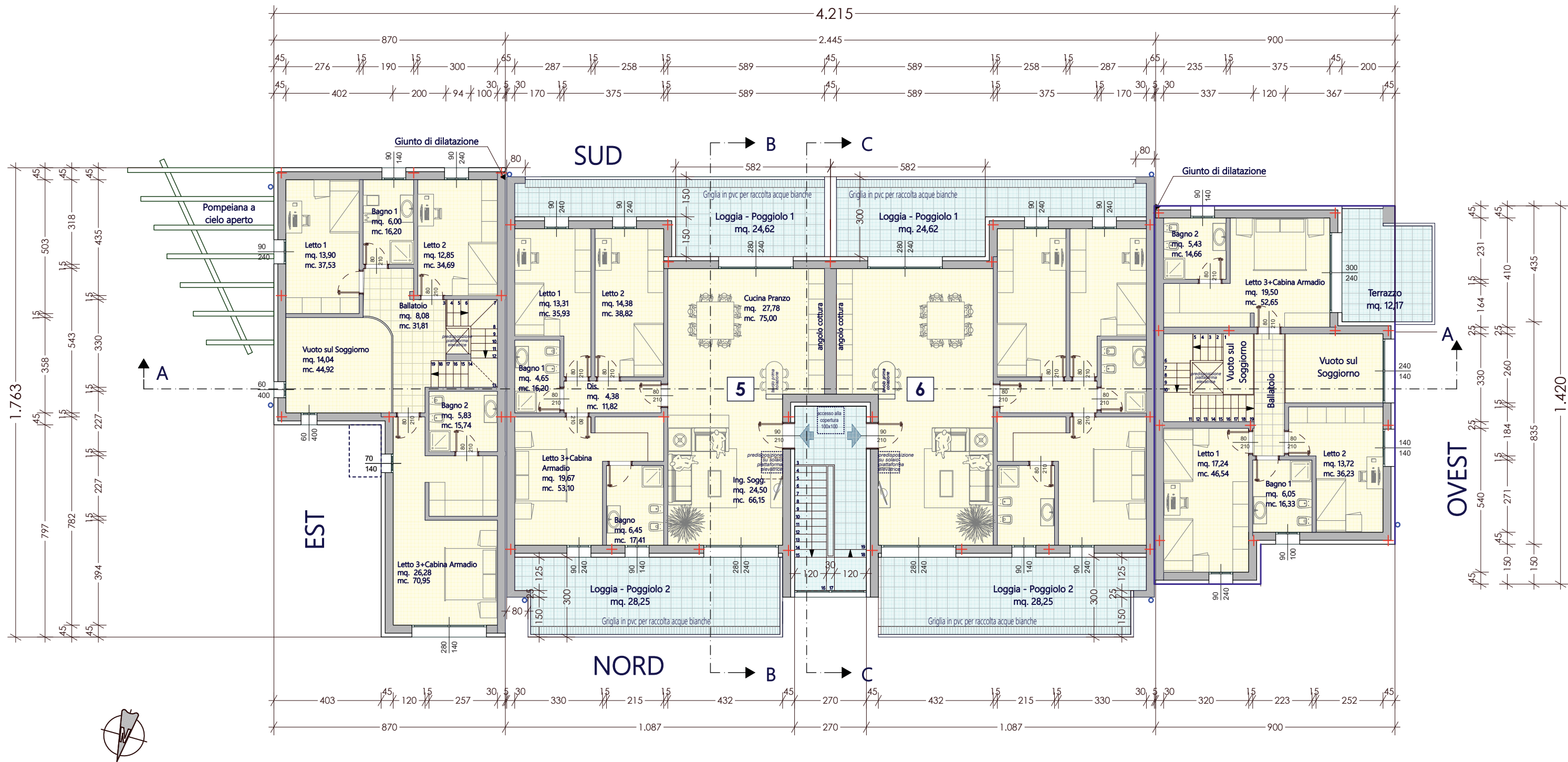
PIANO PRIMO
